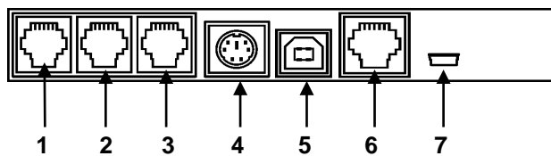
2. ábra - Csatlakozók a pénztárgép alján
